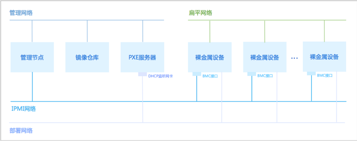
图 32: 裸金属管理网络拓扑
