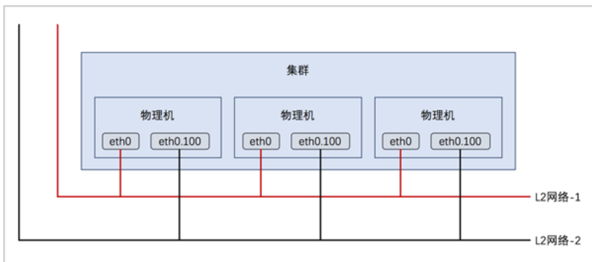
图 14: 二层网络
