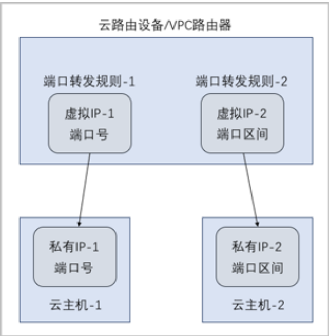
图 23: 虚拟IP-端口转发
