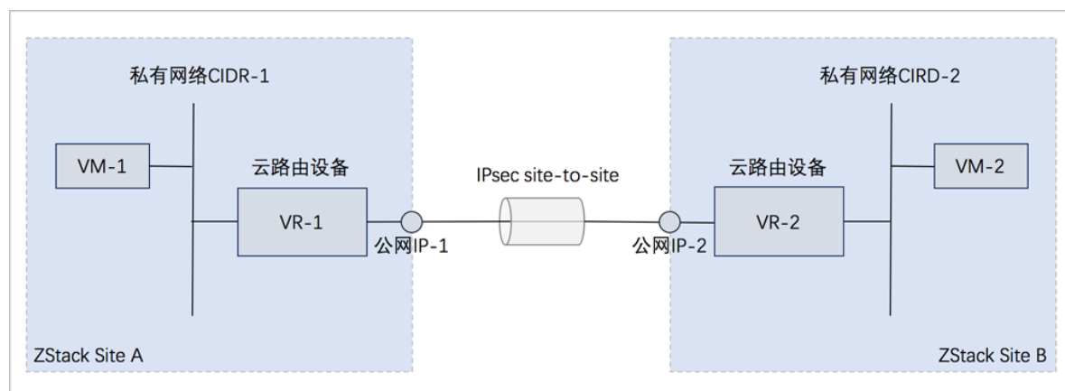
图 25: 云路由网络下IPsec隧道应用场景
