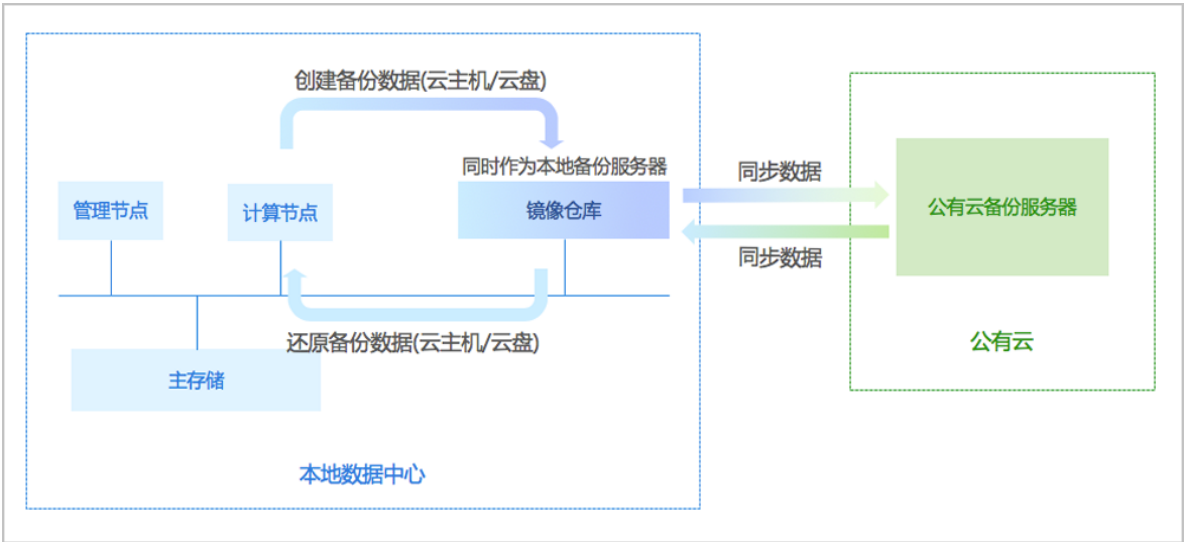
图 37: 公有云灾备场景1
