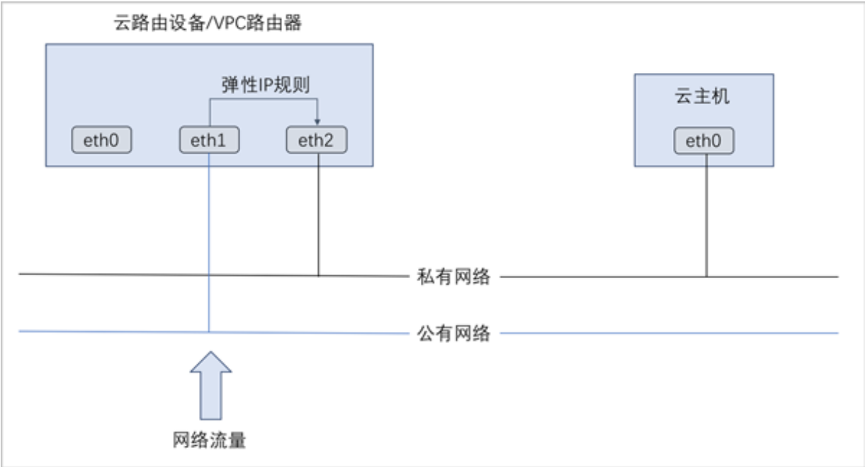
图 21: 云路由网络/VPC下弹性IP的应用场景
