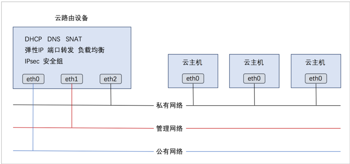
图 16: 部署方式-2
